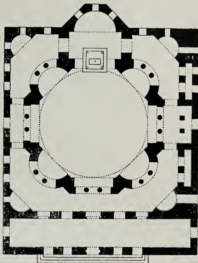
Figura 42 —Planta de la iglesia de los Santos Sergio y Baco en Constantinopla.
